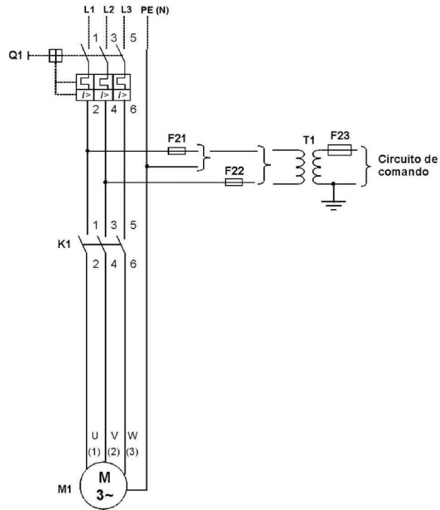
Circuito de potência
