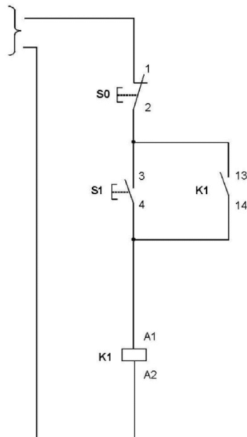
Circuito de comando
