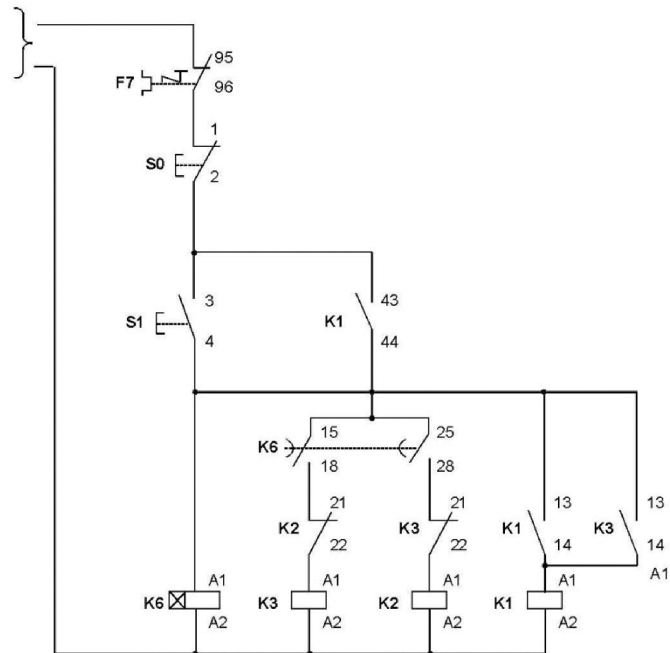
Circuito de comando
